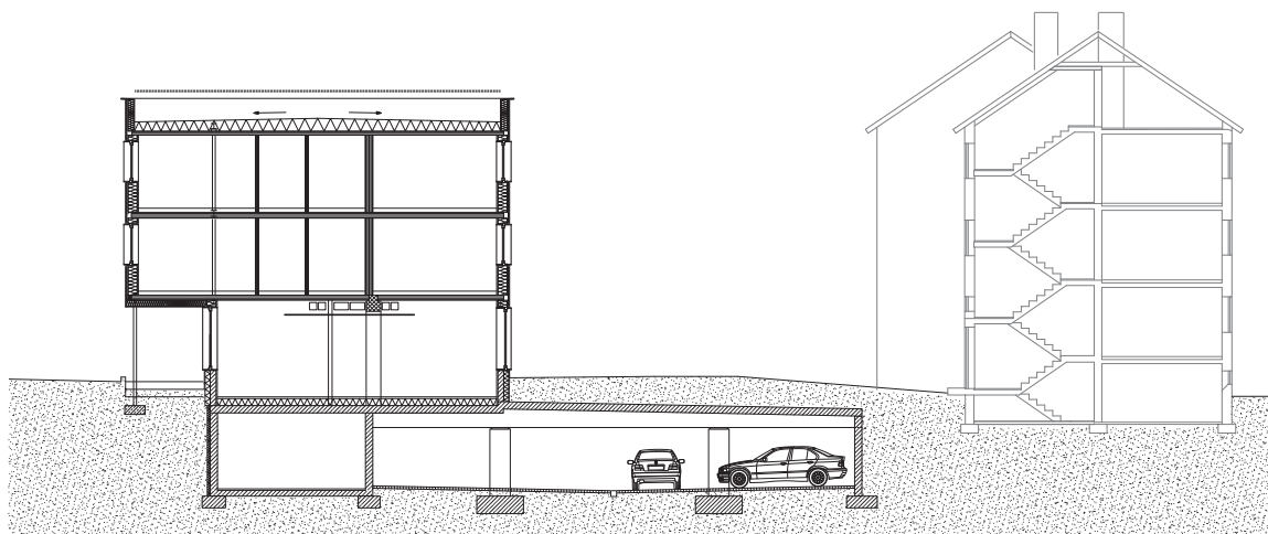
Querschnitt, Neubau
