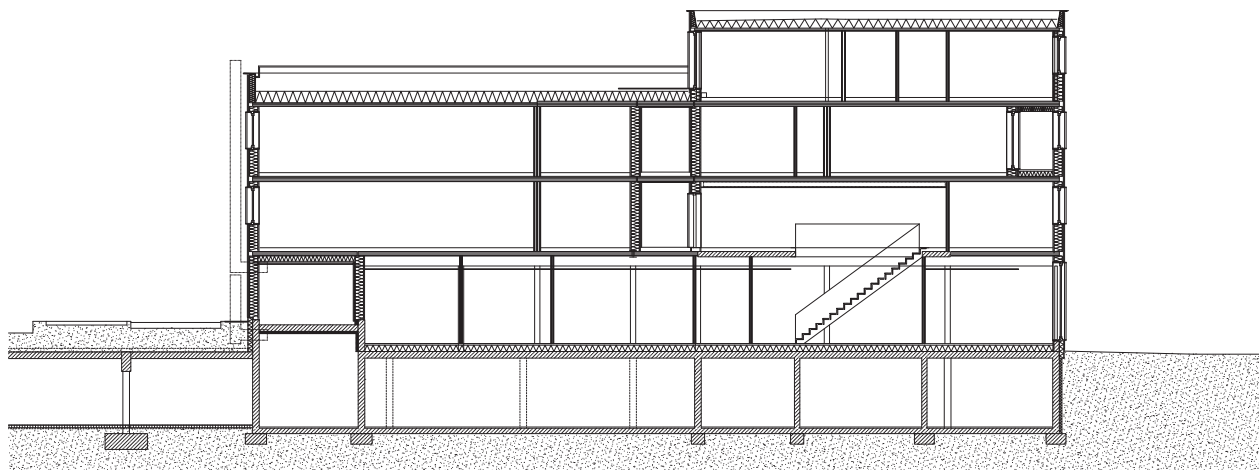
Längsschnitt, Neubau
