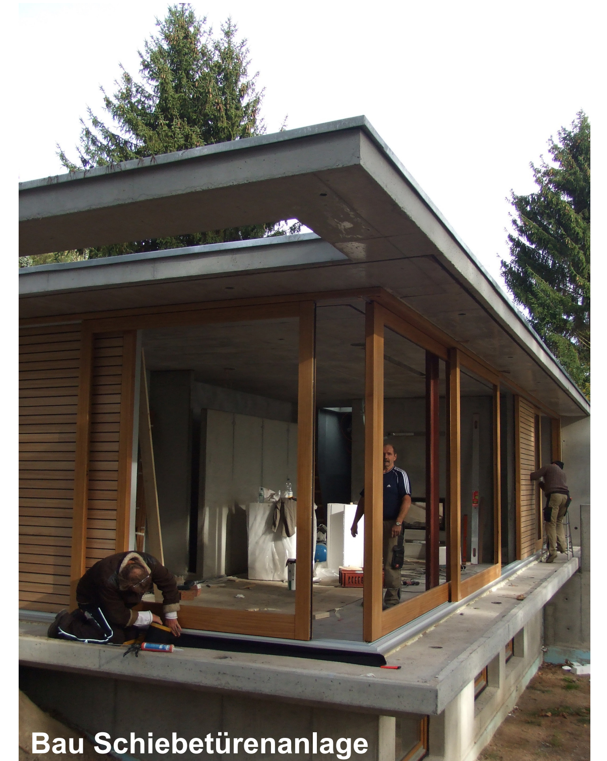
Bau Schiebetürenanlage
